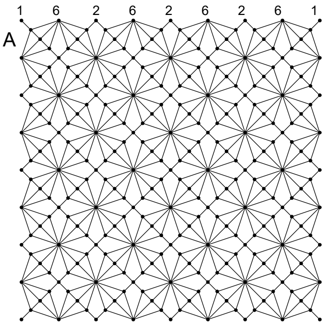
6-paarige Verbindungen ("Sternchen")
